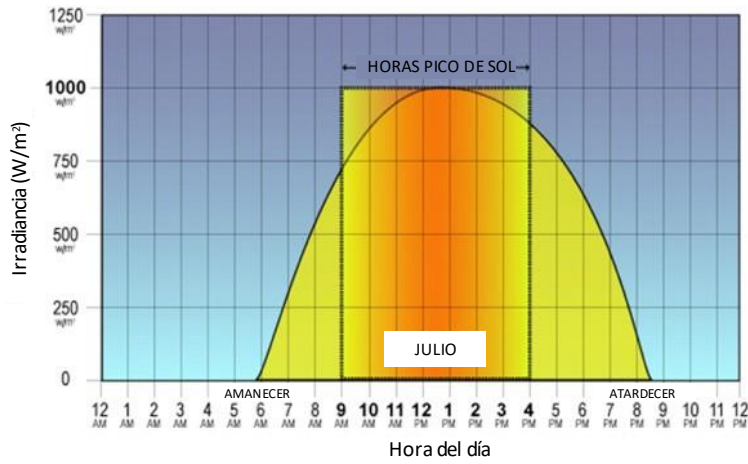
Figura 2.5.1.a: Irradiación solar basada en la hora del día
